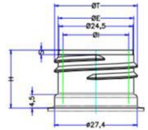
DETALHE DO GARGALO ESCALA 2:1
