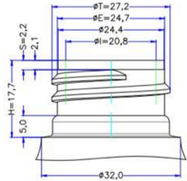
DETALHE DO GARGALO ESCALA 3 : 1
