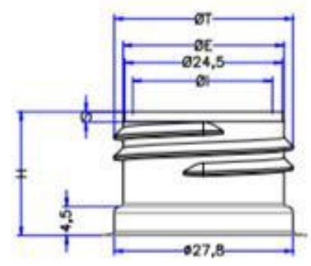
DETALHE DO GARGALO ESCALA 2:1
