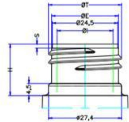
DETALHE DO GARGALO ESCALA 2:1
